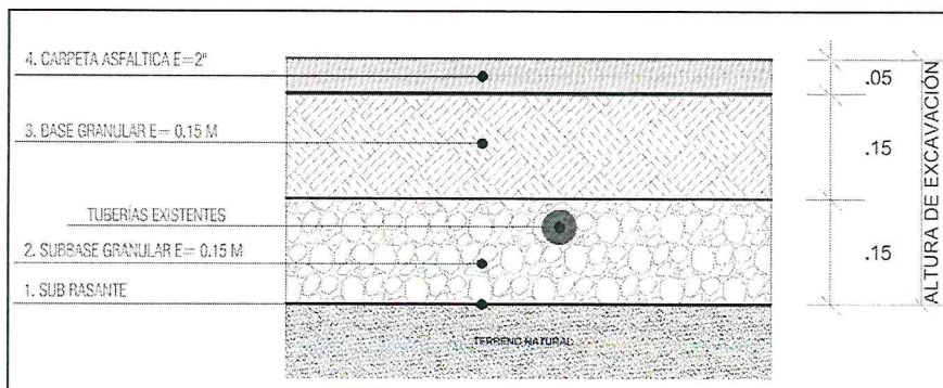
Imagen 02: Propuesta de profundizar la tubería de agua
